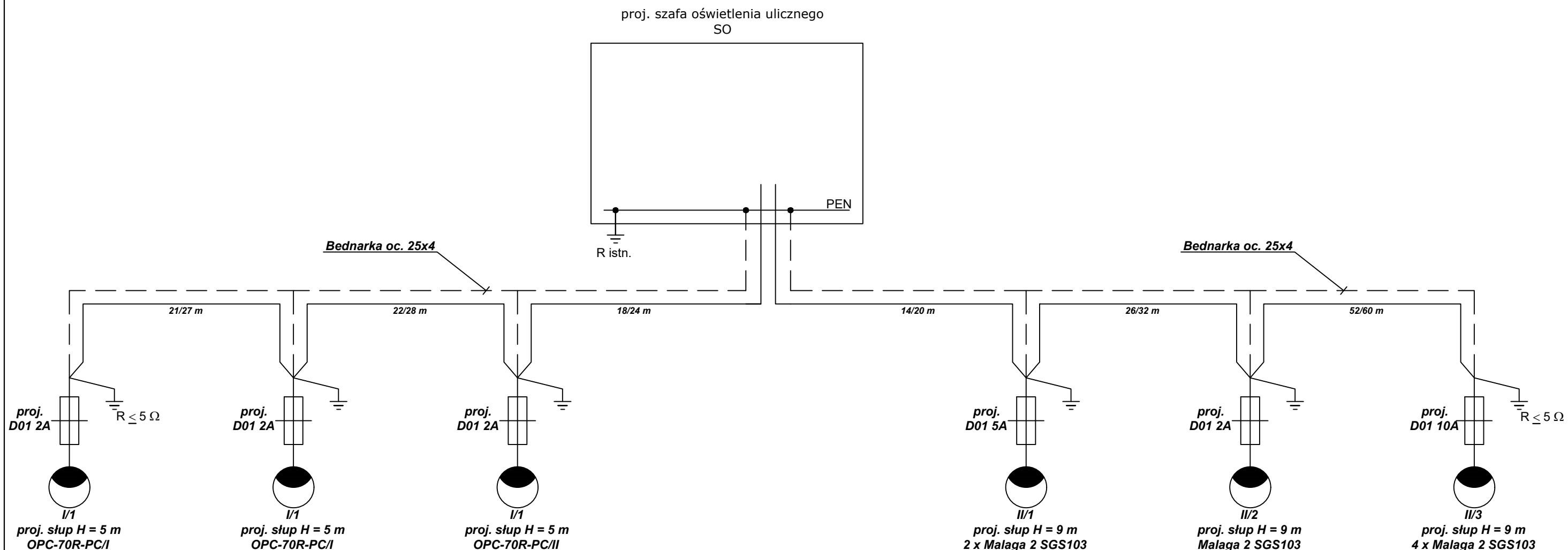
proj. obw. nr I, YAKY 4x25 mm 2
