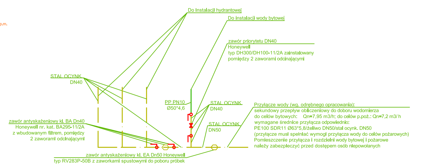
SCHEMAT ROZDZIAJU INSTALACJI WODY NA CELE BYTOWE I PRZECIWPÓZAROWE PO WEJŚCIU PRZYŁĄCZA WODY DO BUDYNKU
