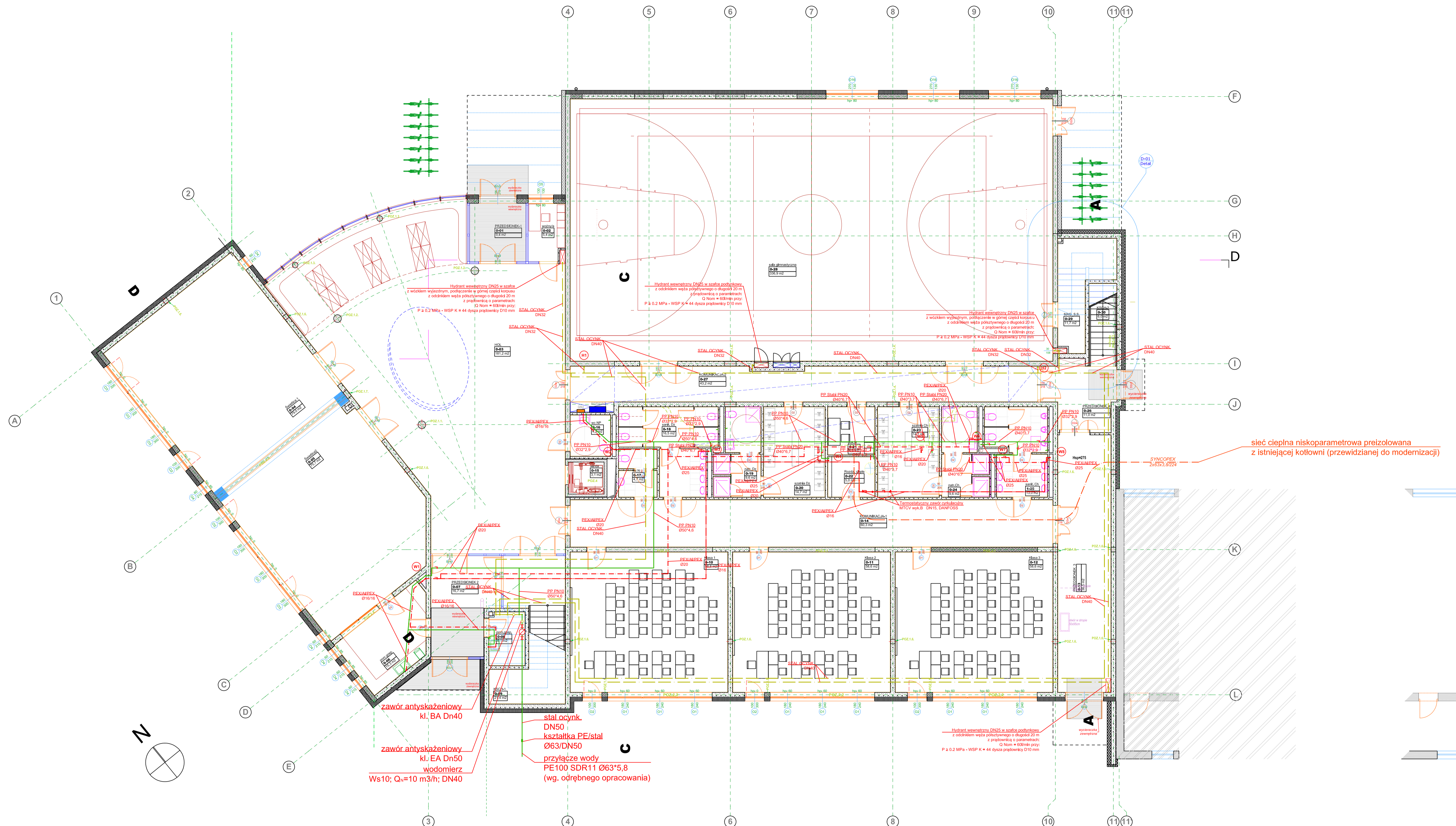
SCHEMAT ROZDZIAJU INSTALACJI WODY NA CELE BYTOWE I PRZECIWPÓZAROWE PO WEJŚCIU PRZYŁĄCZA WODY DO BUDYNKU
