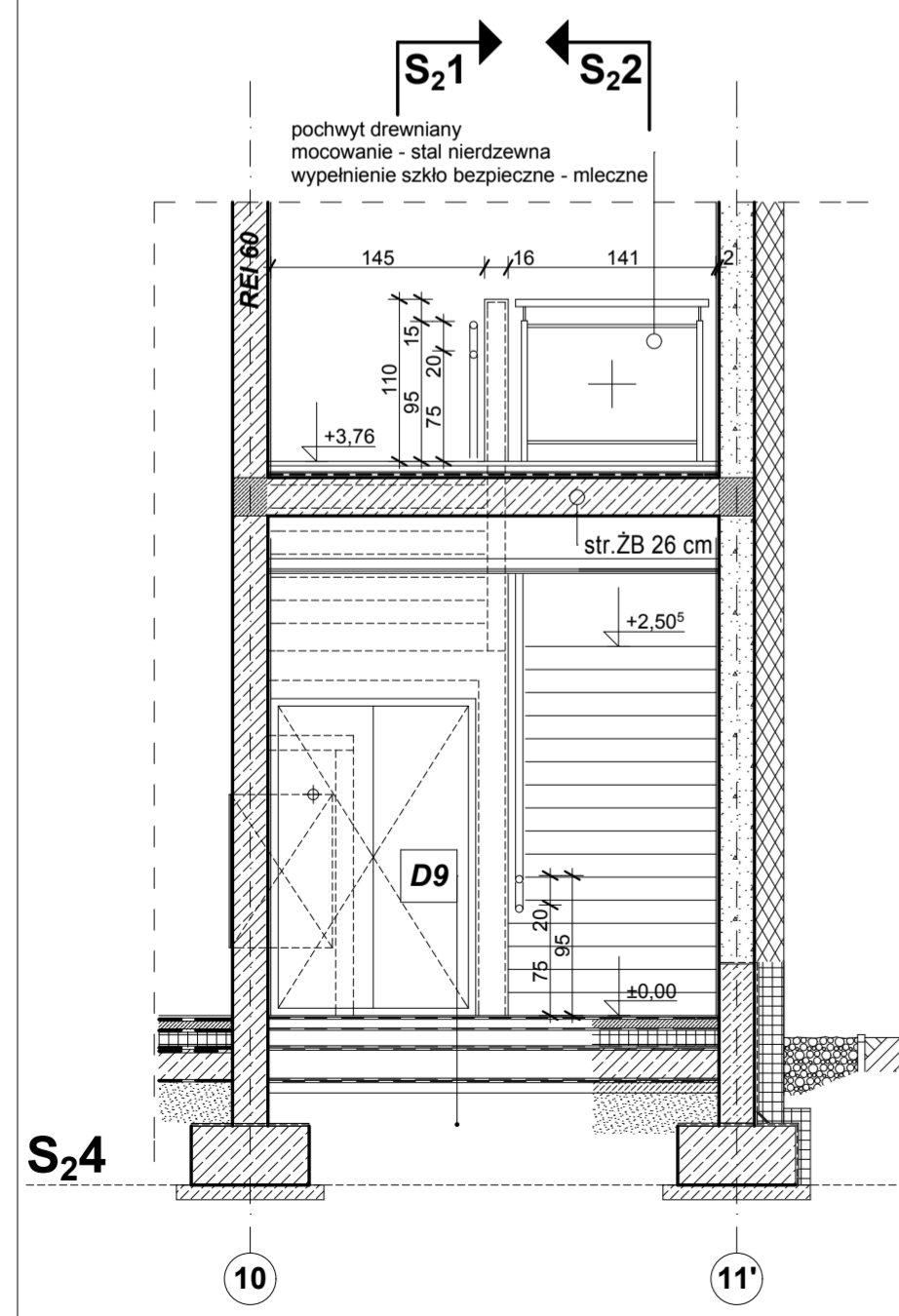
SCHODY_2 1. PIĘTRO
