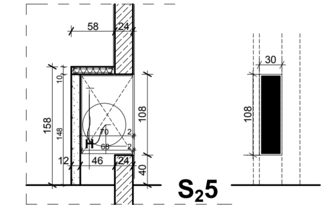
PRZEKRÓJ PRZEZ OBUDOWĘ HYDRANTU
