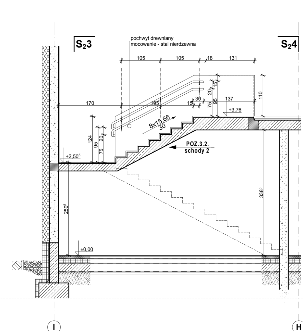
SCHODY_2 PARTER
