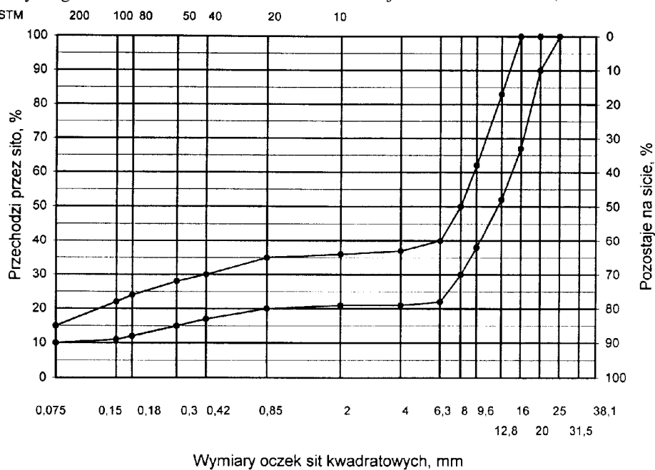
Rys. 5. Krzywe graniczne uziarnienia mieszanki mineralnej BA od 0 do 20 mm (mieszanka o nieciągłym uziarnieniu)
