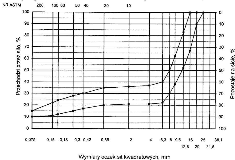
Rys. 5. Krzywe graniczne uziarnienia mieszanki mineralnej BA od 0 do 20 mm (mieszanka o nieciąglym uziarnieniu)
