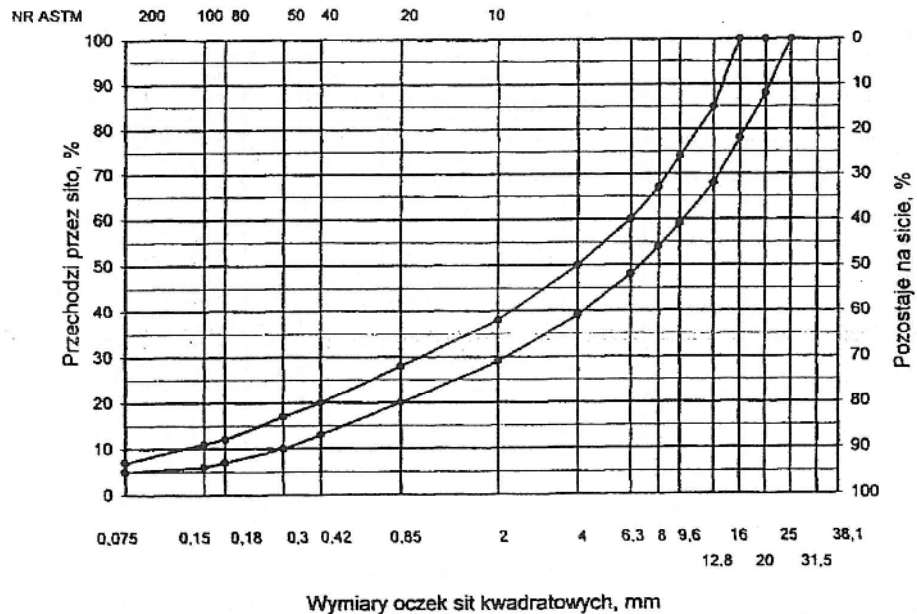
Rys. 4. Krzywe graniczne uziarnienia mieszanki mineralnej BA od 0 do 20 mm do warstwy ściaralnej nawierzchni drogi o obciążeniu ruchem od KR3 do KR6
