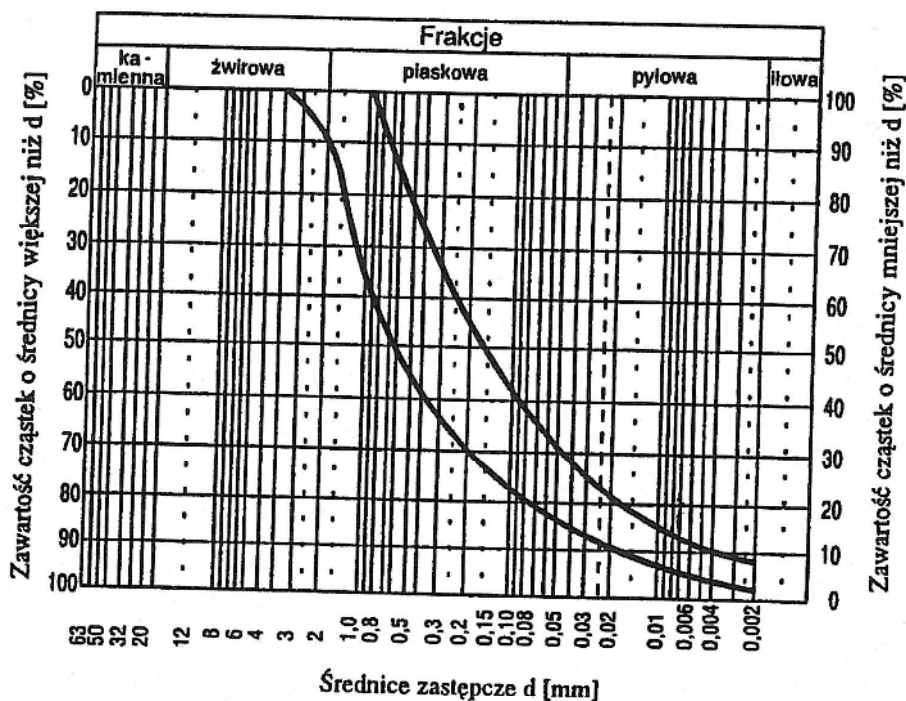
Rys. 1. Obszar uziarnienia optymalnej mieszanki gliniasto-piaskowej
