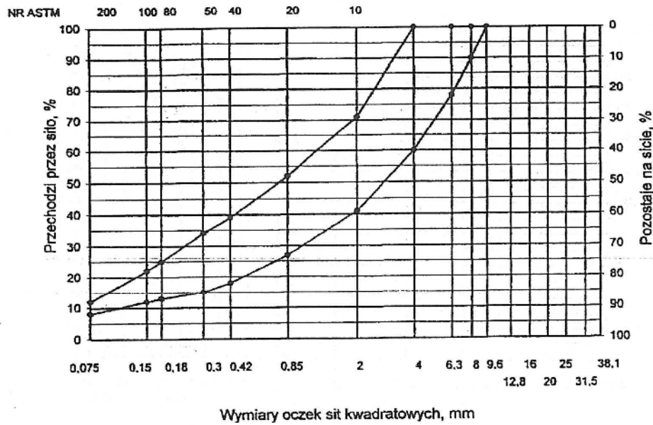
Rys. 3. Krzywe graniczne uziarnienia mieszanki mineralnej BA od 0 do 8 mm, od 0 do 6,3 mm do warstwy ściaralnej nawierzchni drogi o obciążeniu ruchem nawierzchni drogi o obciążeniu ruchem KR1 lub KR2
