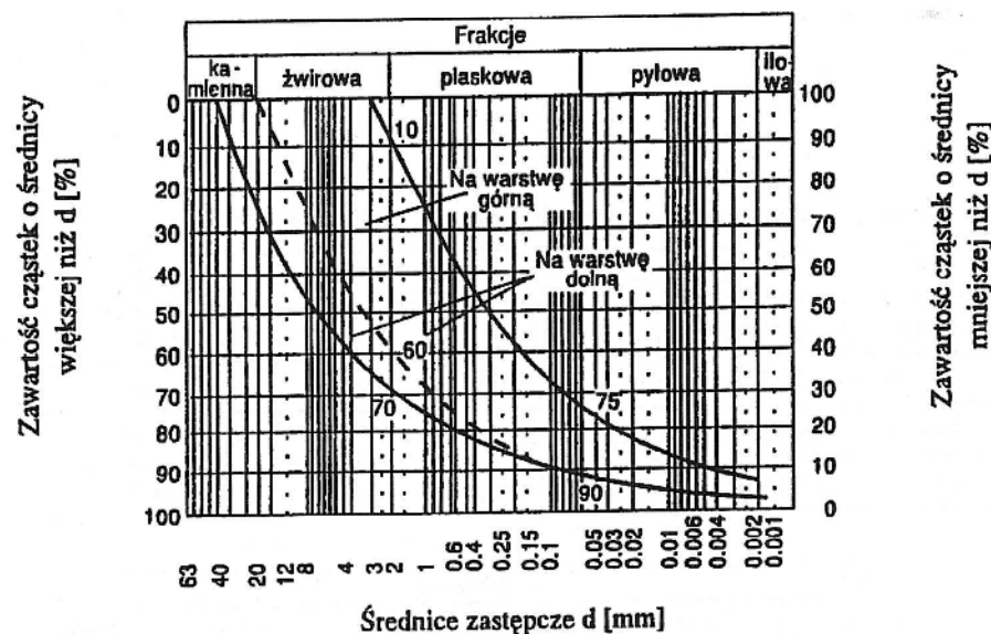
Rys. 2. Obszar uziarnienia optymalnej mieszanki gliniasto-żwirowej
