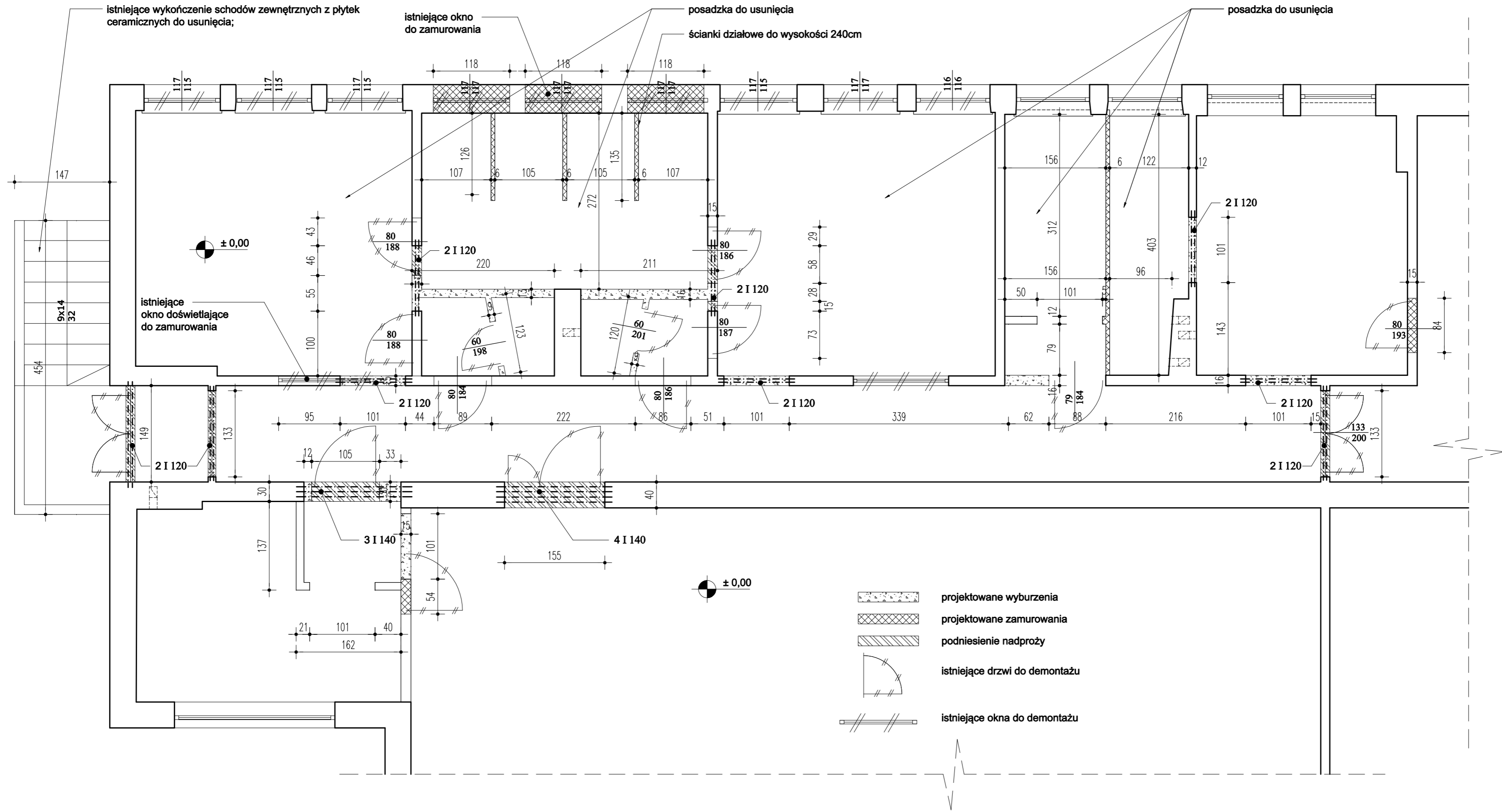
R RZUT ZAPLECZA ISTNIEJĄCEJ SALI GIMNASTYCZNEJ Skala 1:50
