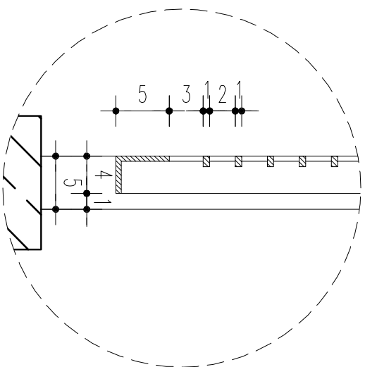
D1 Detal typowego przesłania Skala 1:5
