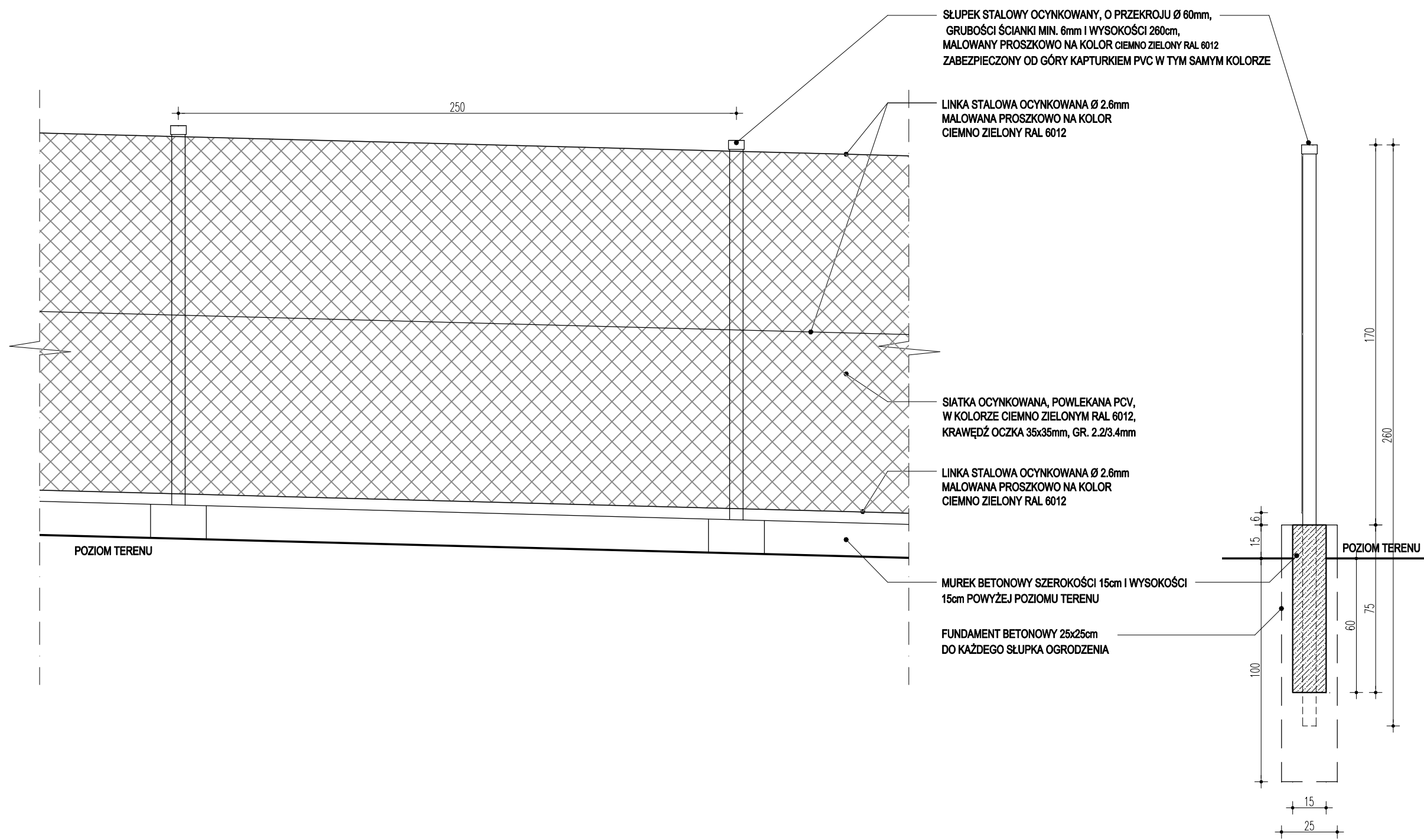
D1 Widok typowego przęsła Skala 1:20
