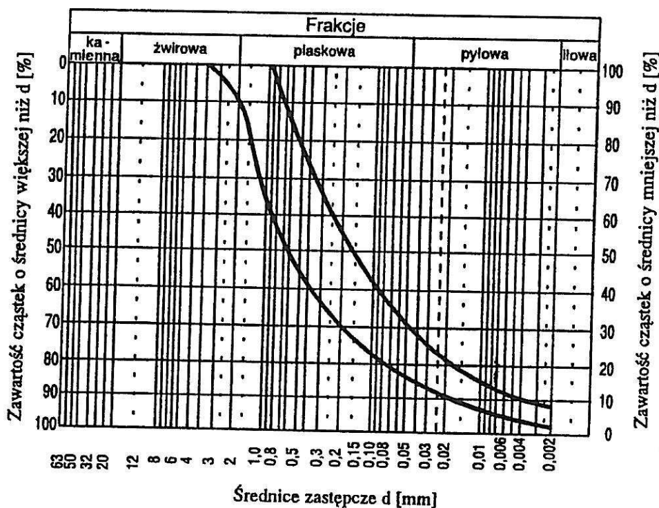
Rys. 1. Obszar uziarnienia optymalnej mieszanki gliniasto-piaskowej
