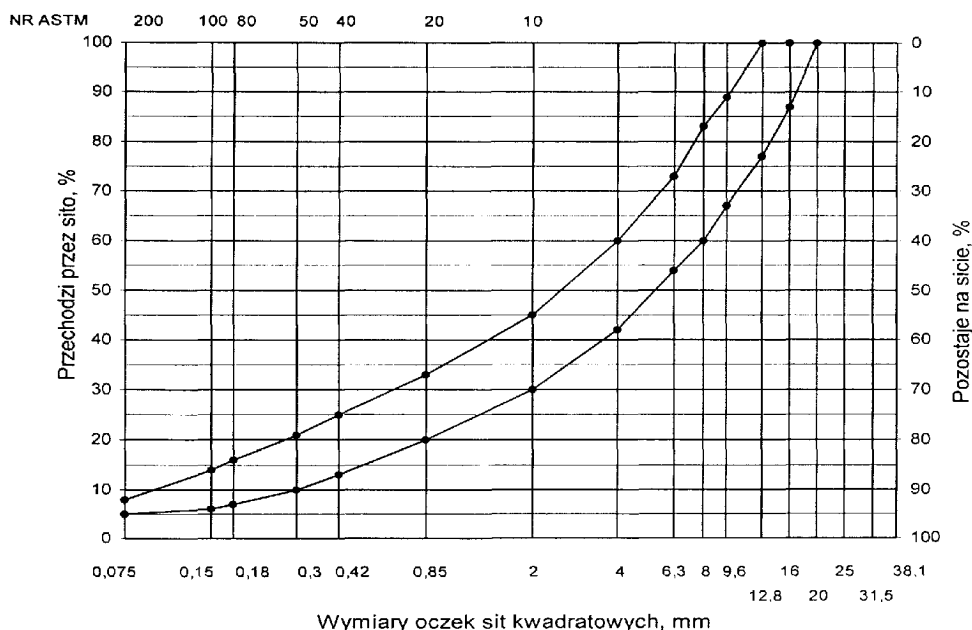
Rys. 2. Krzywe graniczne uziarnienia mieszanki mineralnej BA od 0 do 16 mm do warstwy wyrównawczej
