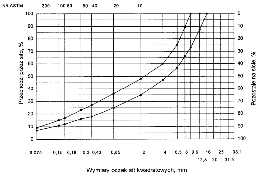
Rys. 1. Krzywe graniczne uziarnienia mieszanki mineralnej BA od 0 do 12.8mm do warstwy ścieralnej
