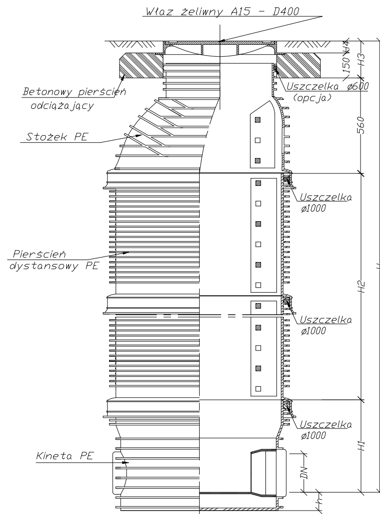
Studzienka kanalizacyjna TEGRA 1000
