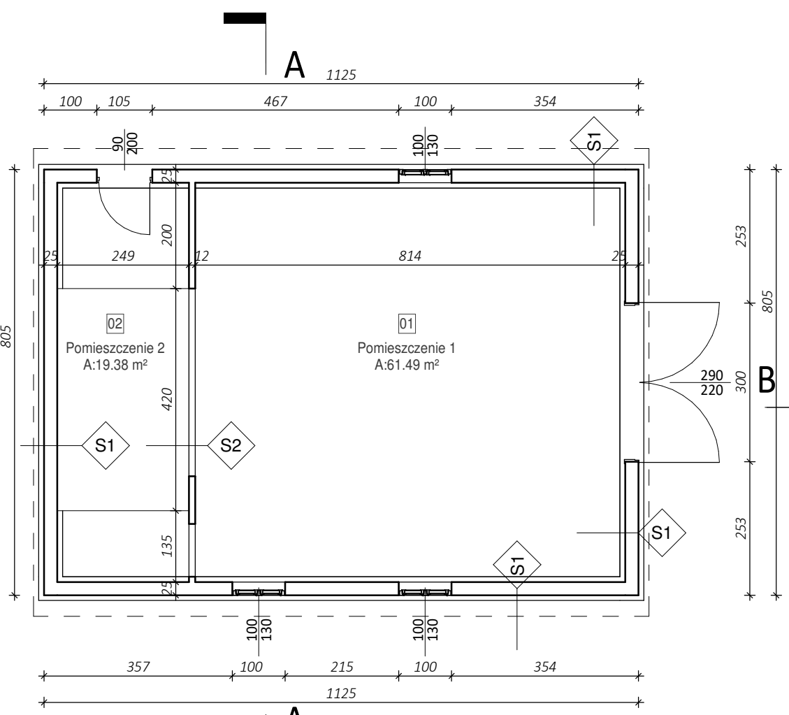
RZUT PARTERU 1 : 100
