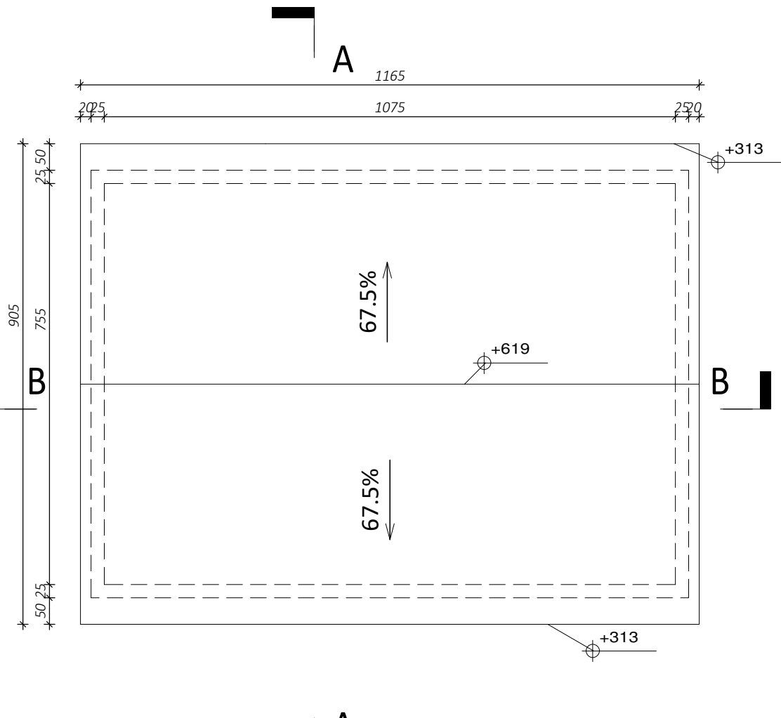
RZUT DACHU 1 : 100
