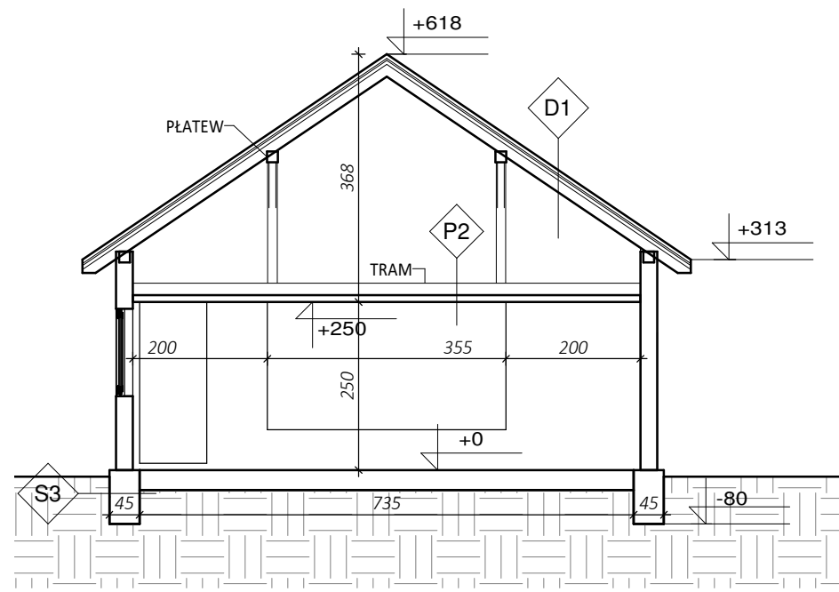
Przekrój A-A 1 : 100
