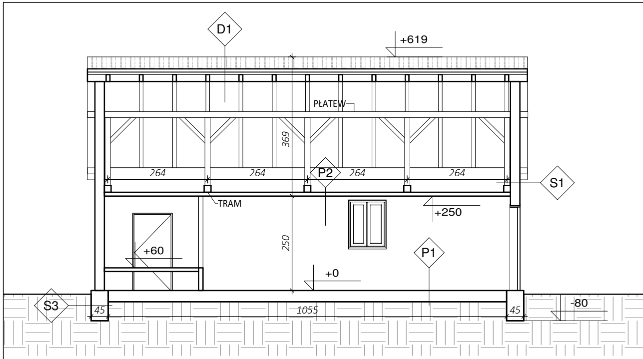
Przekrój B-B 1 : 100
