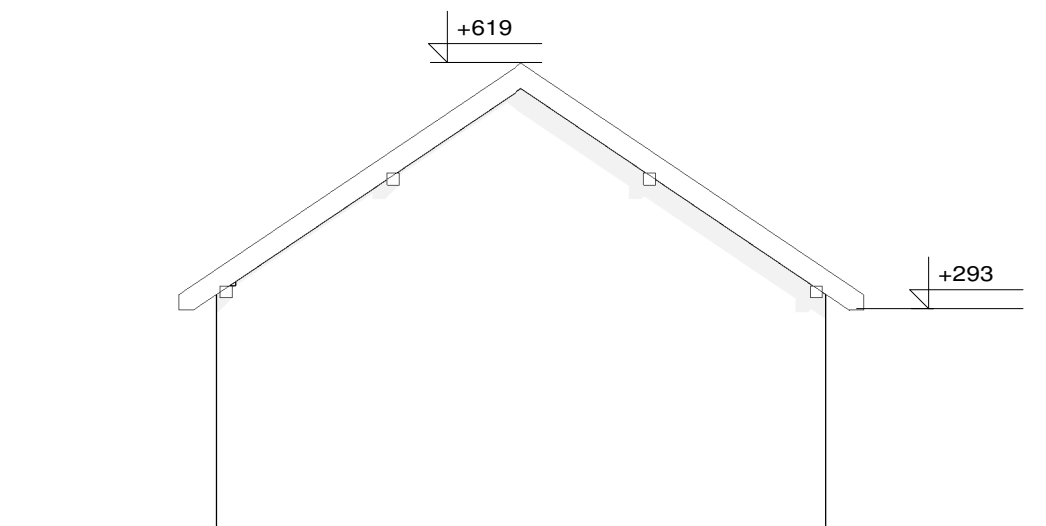
Elewacja Północno - Zachodnia 1 : 100
