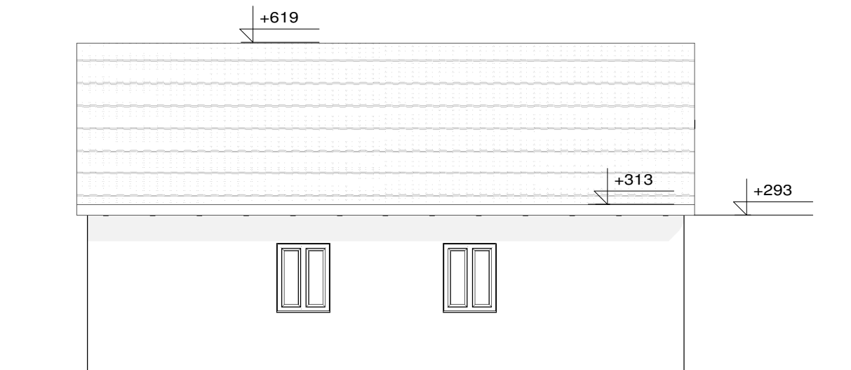
Elewacja Południowo - Zachodnia 1 : 100
