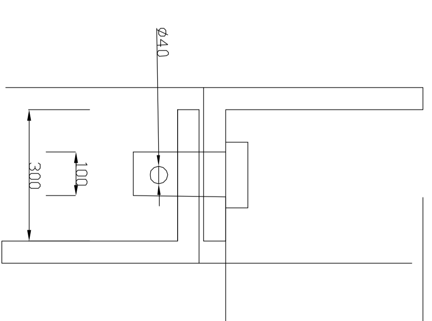
ZAWIAS SZCZEGÓL "A"
