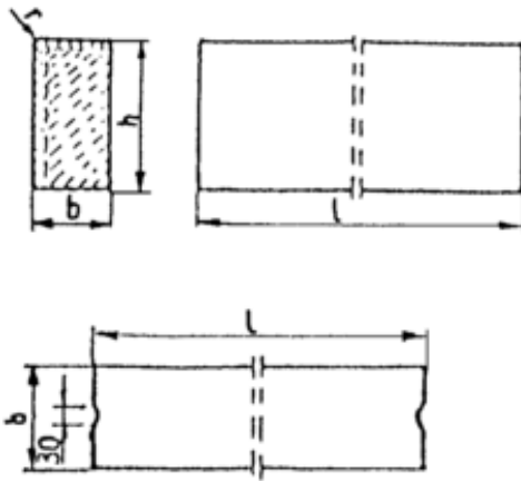
Rys. 1. Wymiarowanie krawężników
