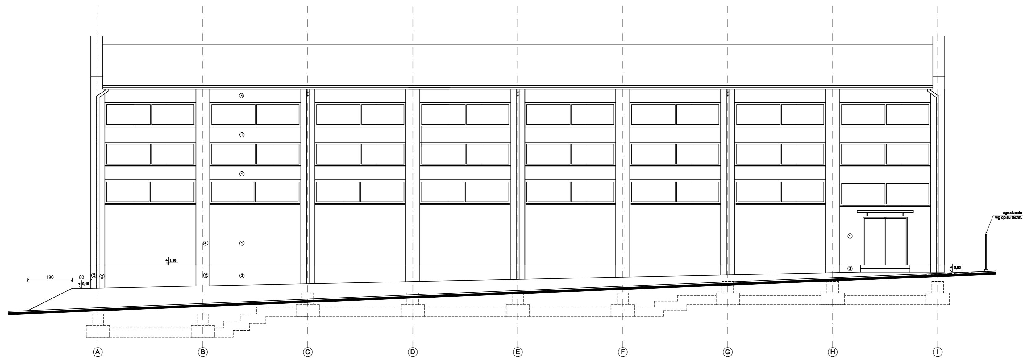
PRZEKRÓJ D-D - ELEWACJA ZACHODNIA
