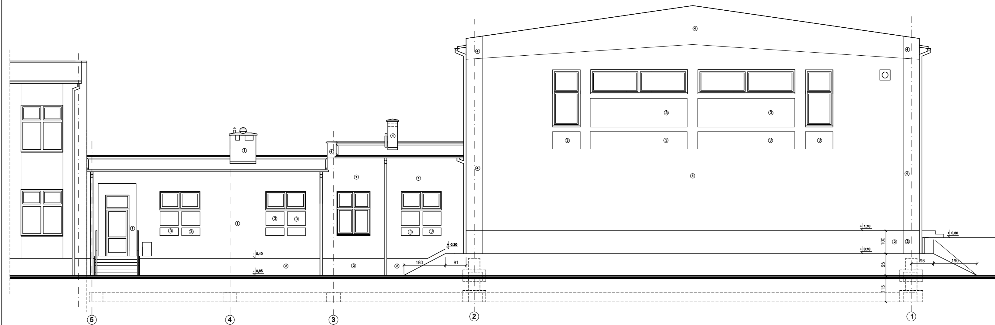
PRZEKRÓJ C-C - ELEWACJA PÓŁNOCNA
