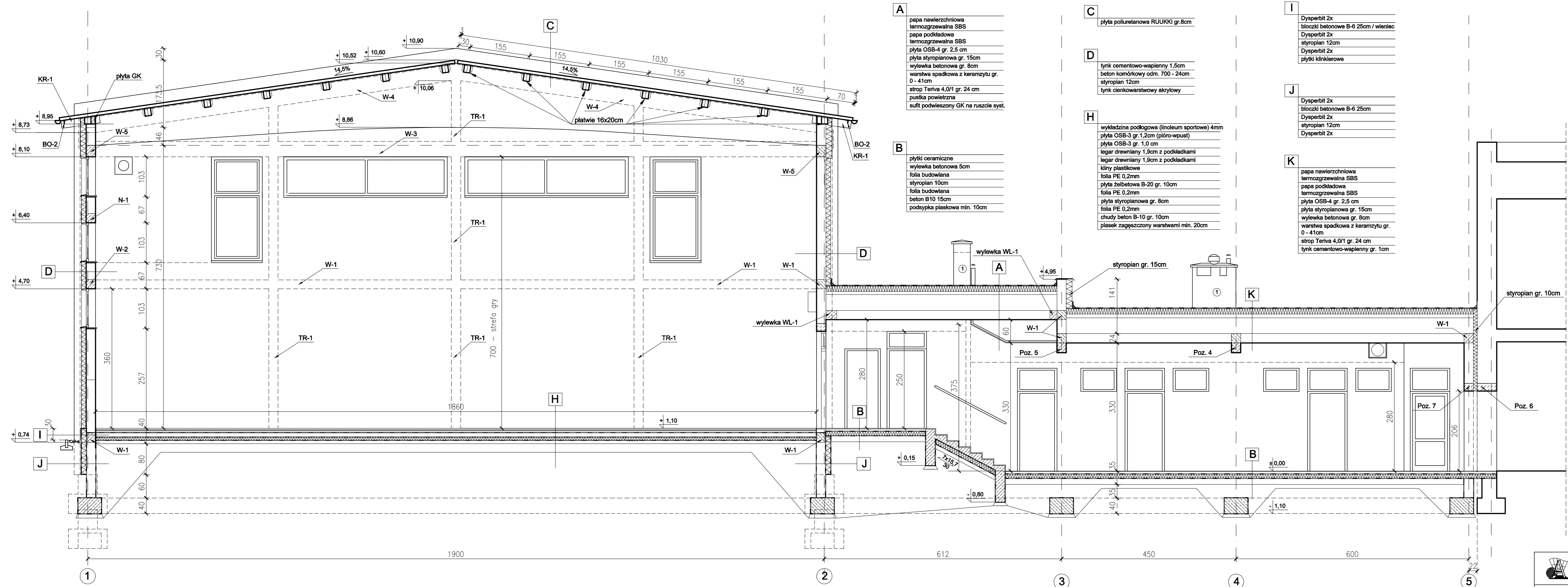
PRZEKRÓJ B-B
