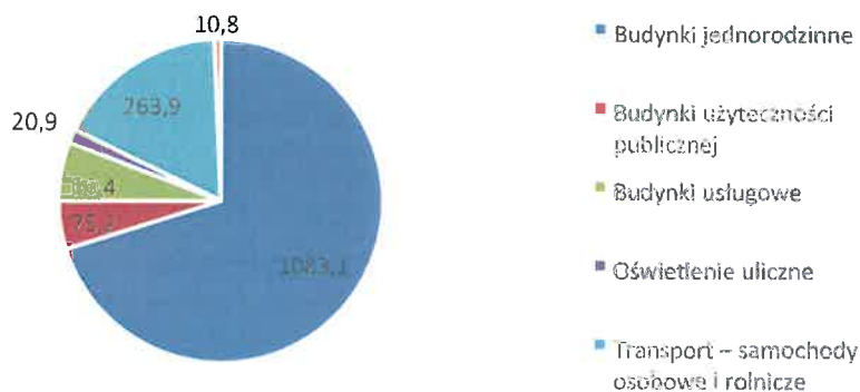
Zbiorcze zestawienie redukcji emisji zanieczyszczeń w poszczególnych obszarach, tCO 2 /rok
