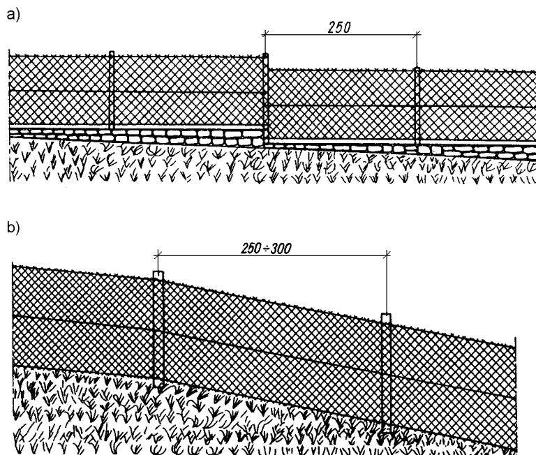
Rys. 6. Przykład ustawienia ogrodzenia siatkowego na terenie pochylonym (wg [6]) 1. Ogrodzenie ze stopniami wysokości 25±30 cm (przy spadku terenu od 1:16 do 1:30) 2. Ogrodzenie równoległe do terenu
