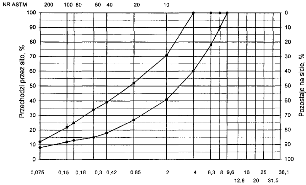
Wymiary oczek sit kwadratowych, mm Rys. 3. Krzywe graniczne uziarnienia mieszanki mineralnej BA od 0 do 8mm, od 0 do 6,3 mm do warstwy ścieralnej nawierzchni drogi o obciążeniu ruchem nawierzchni drogi o obciążeniu ruchem KR1 lub KR2
