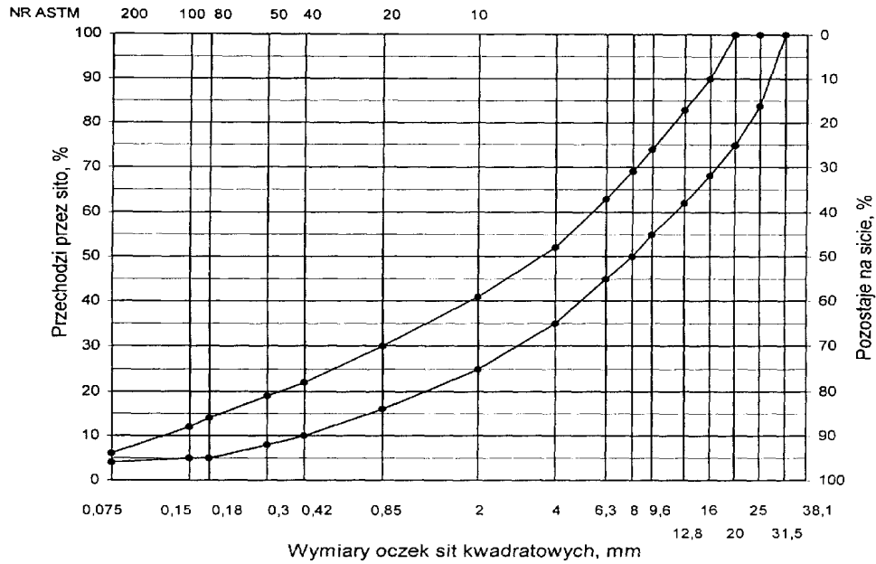
Rys. 11. Krzywe graniczne uziarnienia mieszanki mineralnej BA 0 do 25 mm do warstwy wiążącej, wyrównawczej i wzmacniającej nawierzchni drogi o obciążeniu ruchem od KR3 do KR6
