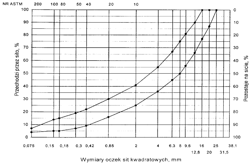
Rys. 12. Krzywe graniczne uziarnienia mieszanki mineralnej BA 0 do 20 mm do warstwy wiążącej, wyrównawczej i wzmacniającej nawierzchni drogi o obciążeniu ruchem od KR3 do KR6
