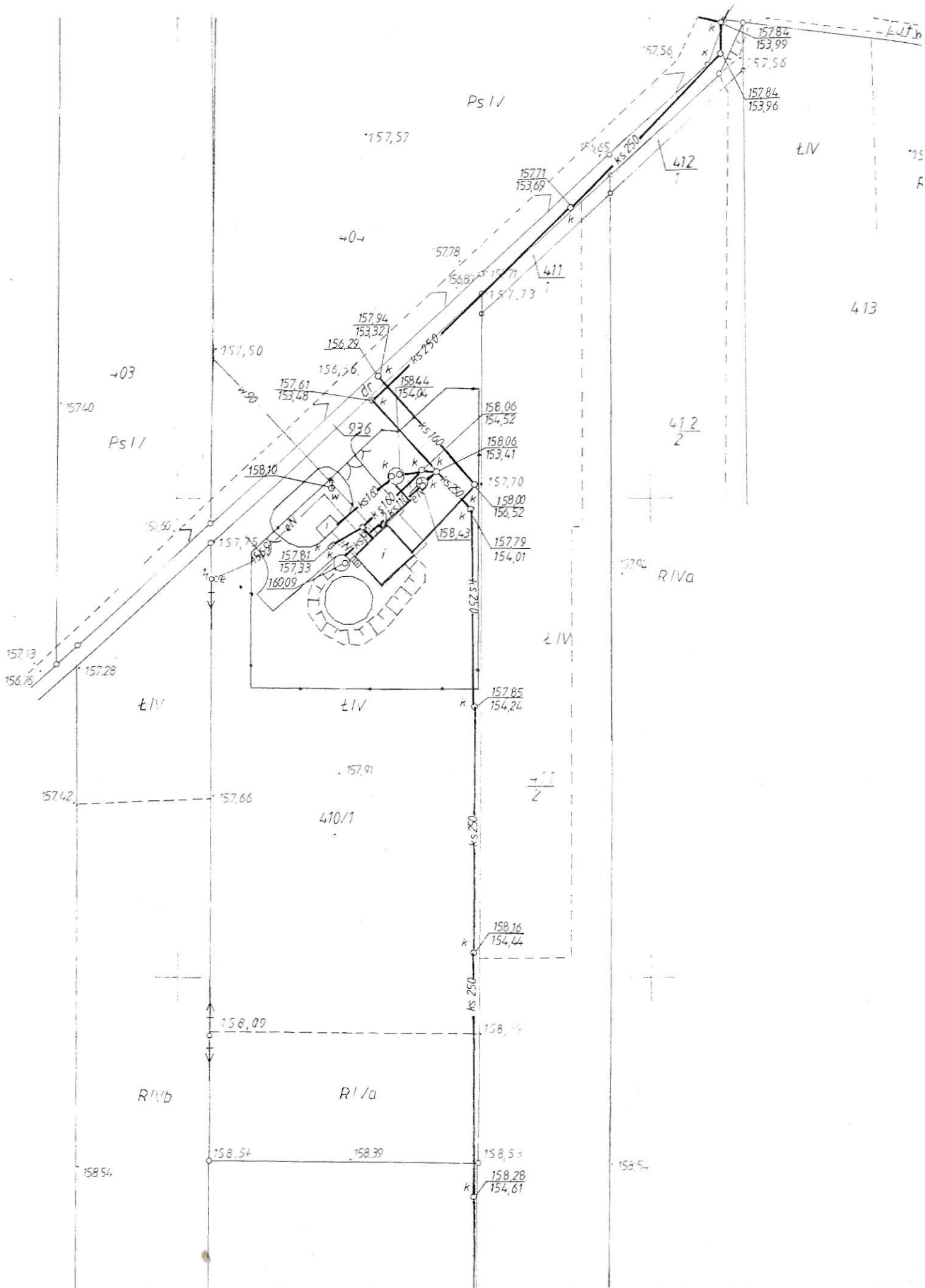
WYRYS Z INWENTARYZACJI OCZYSZCZALNI ŚCIEKÓW W GALEWICACH
