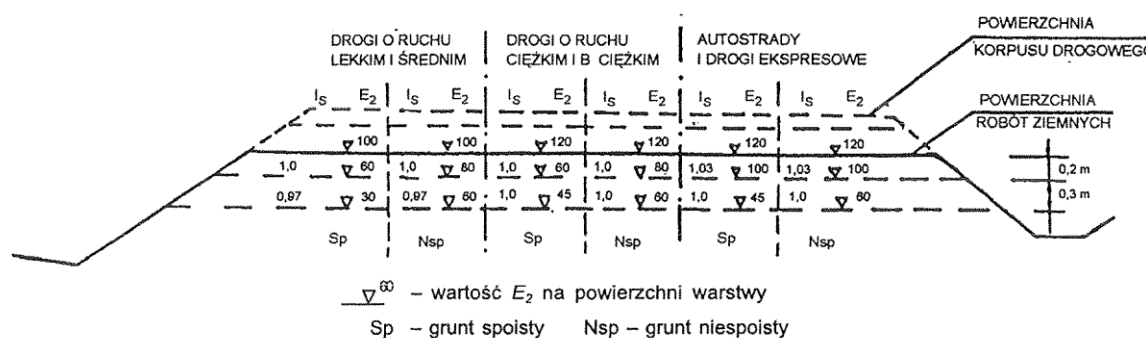
Rysunek 4 – Wartości wymagane w podłożu wykopów: wskaźnika zagęszczenia I_s i wtórny moduł odkształcenia E_2 , megapaskali
