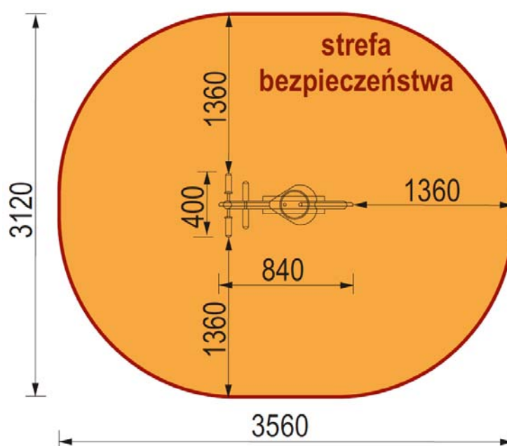
Rys.12 Sprężynowiec rowerek - strefa upadku.
