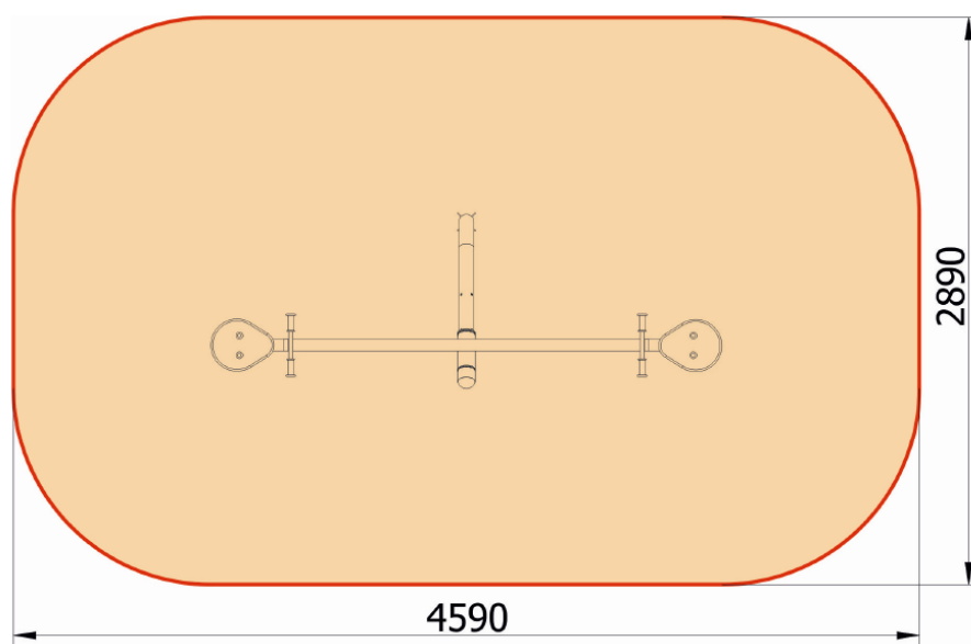
Rys.7 Huśtawka diagonalna / wagowa metalowa - strefa upadku.
