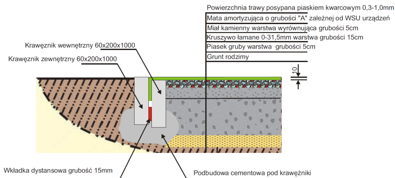
Rys. 21 Przygotowanie podbudowy z piasku i przekrój przez syntetyczną nawierzchnię amortyzującą. (W tym wypadku głębokość wykopu dla nawierzchni amortyzującej upadki z wysokości 1,8m.)
