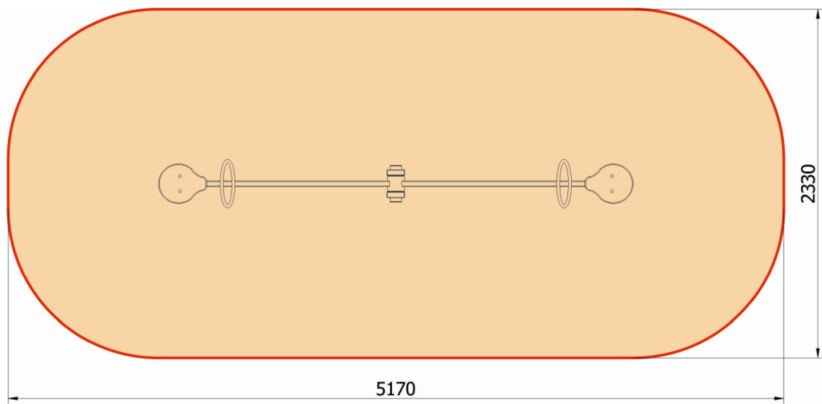
Rys. 5 Huśtawka wagowa duża - strefa upadku.
