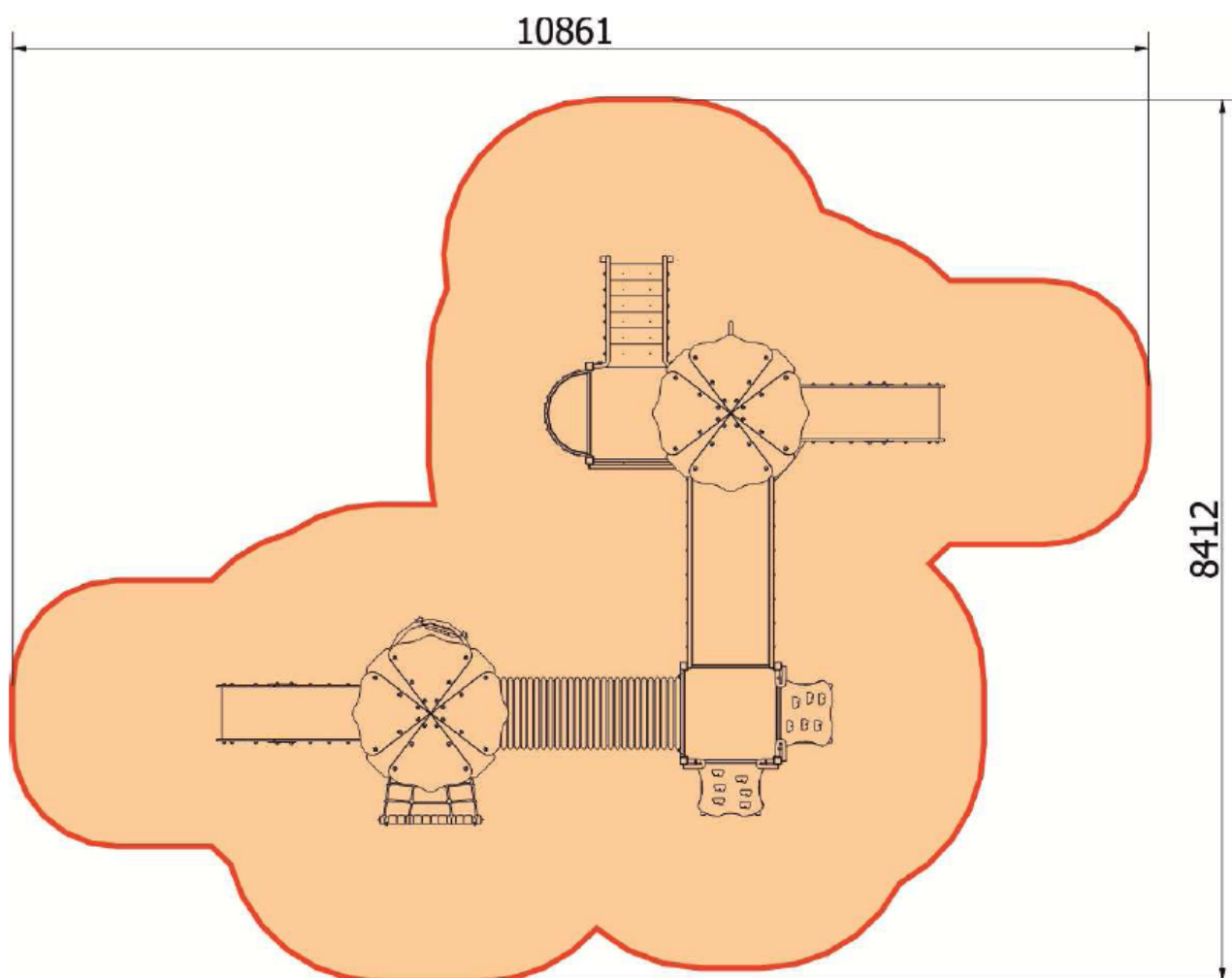
Rys.2 Wymiary i strefa bezpieczeństwa - zestaw zabawowy dwuwieżowy
