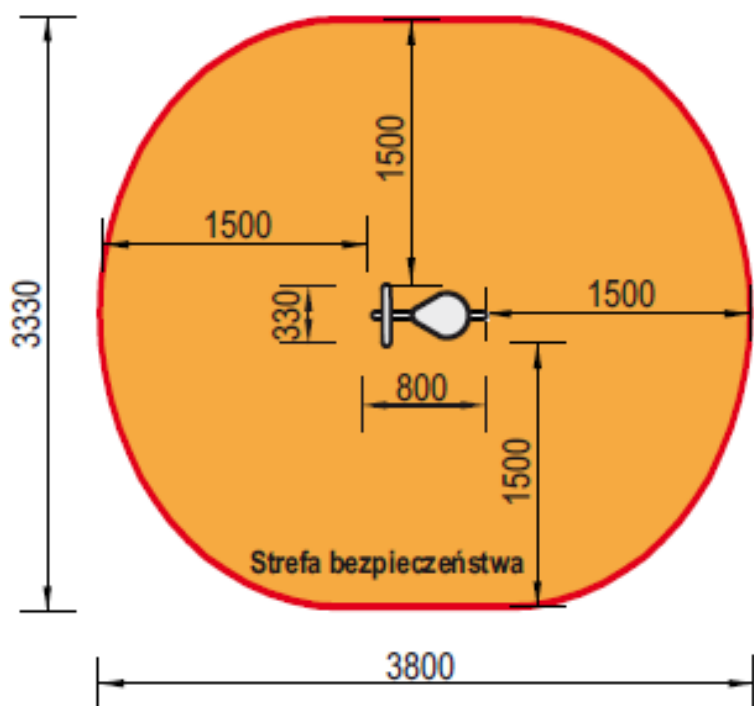
Rys.8 Bujak na sprężynie - rowerek (tu na ilustracji malowany - ale ma być ze stali nierdzewnej )
