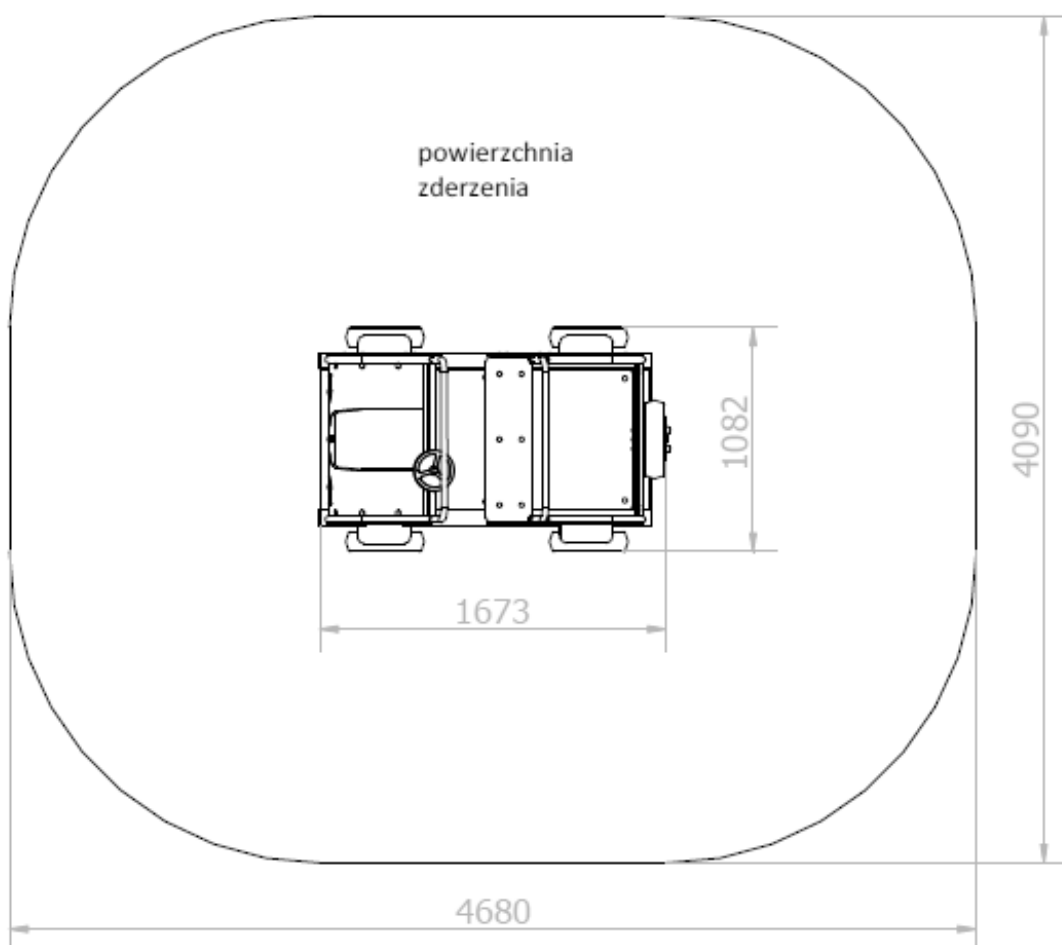
Rys.4 Duży bujak samochód - strefa bezpieczeństwa
