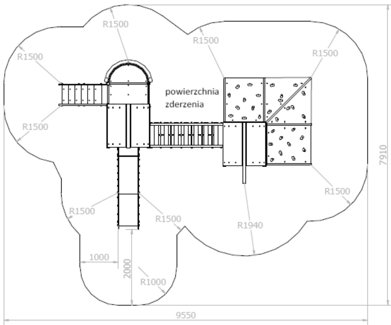
Rys.2 Wymiary i strefa bezpieczeństwa - zestaw zabawowy dwuwieżowy
