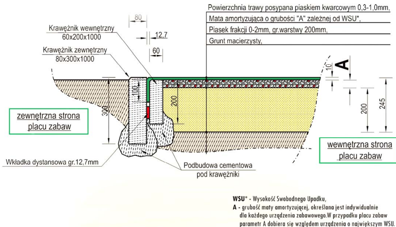
Rys. 18 Przygotowanie podbudowy z piasku i przekrój przez syntetyczną nawierzchnię amortyzującą. (W tym wypadku głębokość wykopu dla nawierzchni amortyzującej upadki z wysokości 1,7m.)
