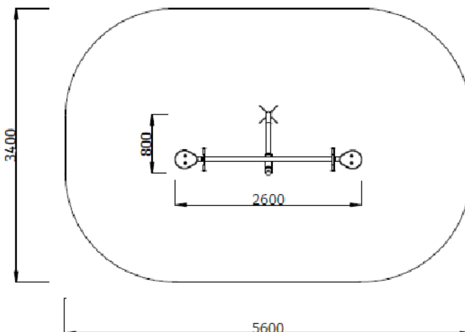
Rys.7 Huśtawka diagonalna / wagowa metalowa - strefa upadku.
