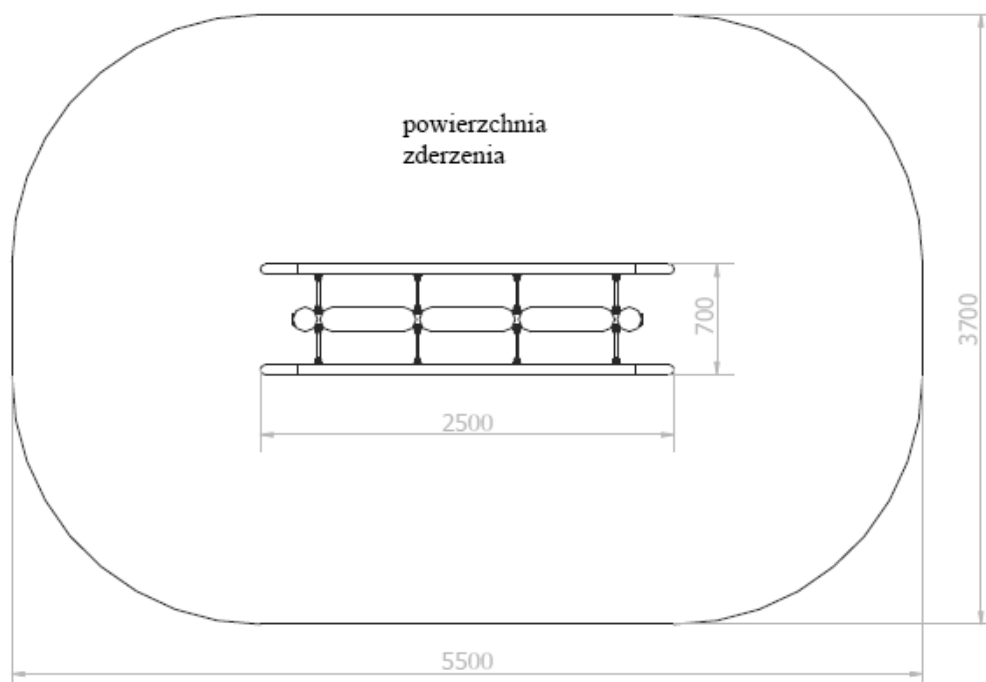
Rys.11 Równoważnia linowa - strefa upadku
