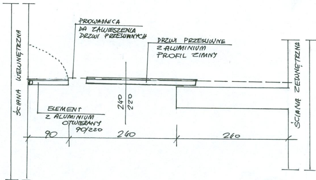
DRZWI PRZESUWNE DO SALI KONFERENCYJNEJ SKALA 1:50
