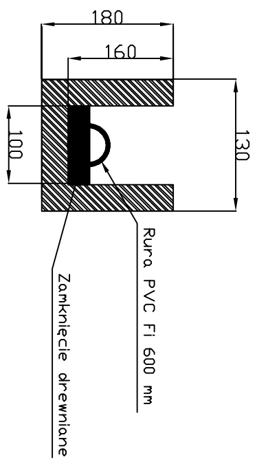
PRZEKRÓJ B - B
