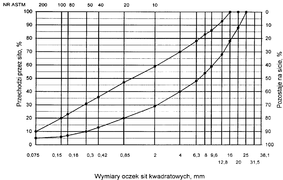
Rys. 1. Krzywe graniczne uziarnienia mieszanki mineralnej BA od 0 do 20 mm do warstwy ścieralnej nawierzchni drogi o obciążeniu ruchem dla KR1
