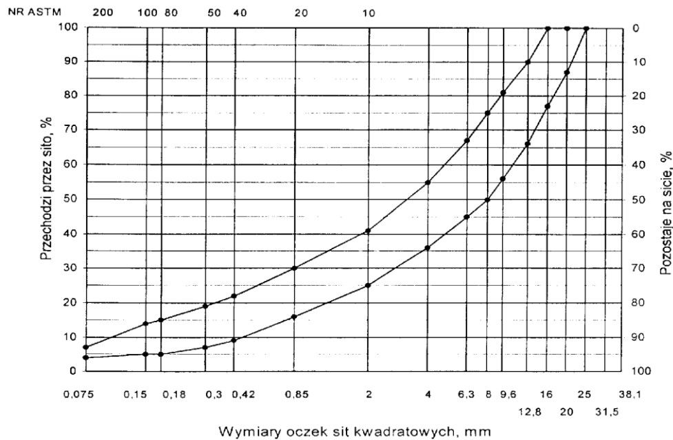
Rys. 12. Krzywe graniczne uziarnienia mieszanki mineralnej BA od 0 do 20 mm do warstwy wiążącej, wyrównawczej i wzmocniającej nawierzchni drogi o obciążeniu ruchem od KR4
