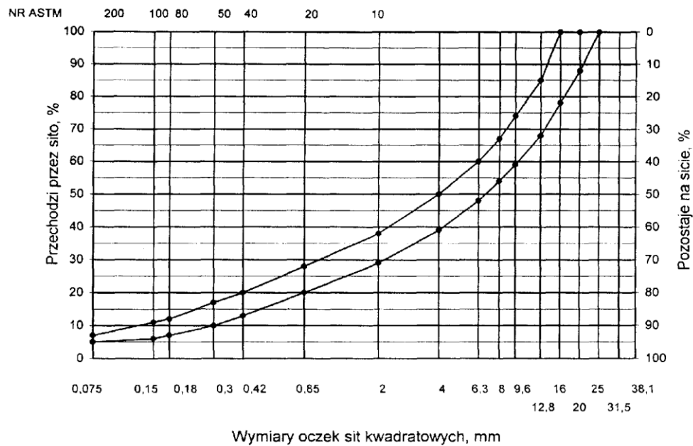
Rys. 4. Krzywe graniczne uziarnienia mieszanki mineralnej BA od 0 do 20 mm do warstwy ścieralnej nawierzchni drogi o obciążeniu ruchem od KR4
