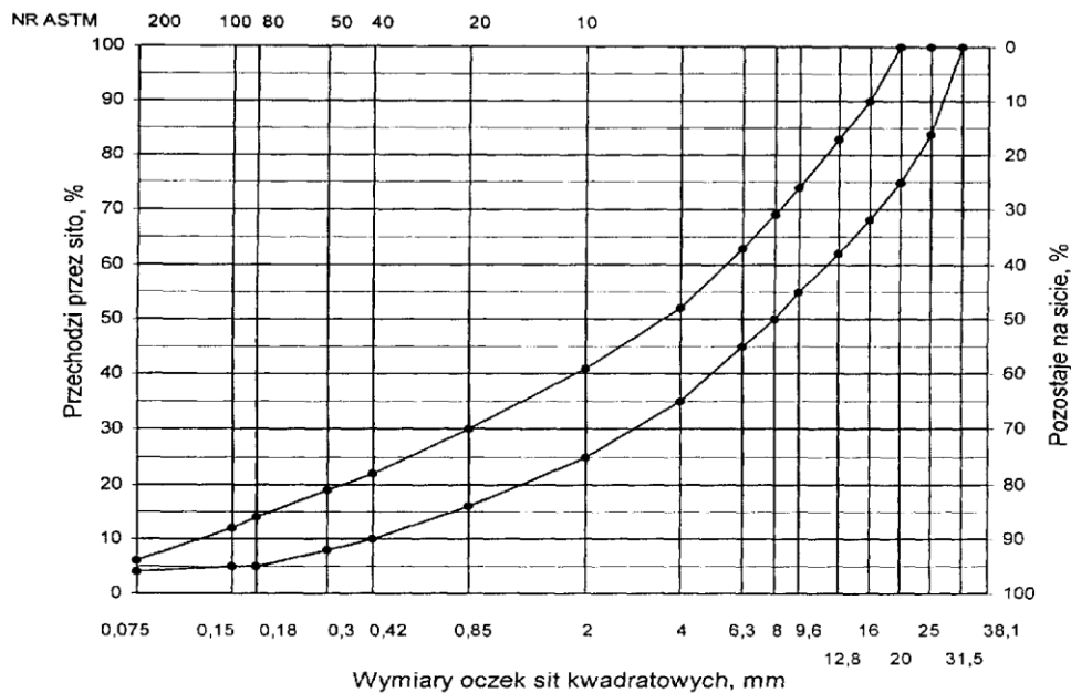
Rys. 11. Krzywe graniczne uziarnienia mieszanki mineralnej BA od 0 do 25 mm do warstwy wiążącej, wyrównawczej i wzmacniającej nawierzchni drogi o obciążeniu ruchem od KR4
