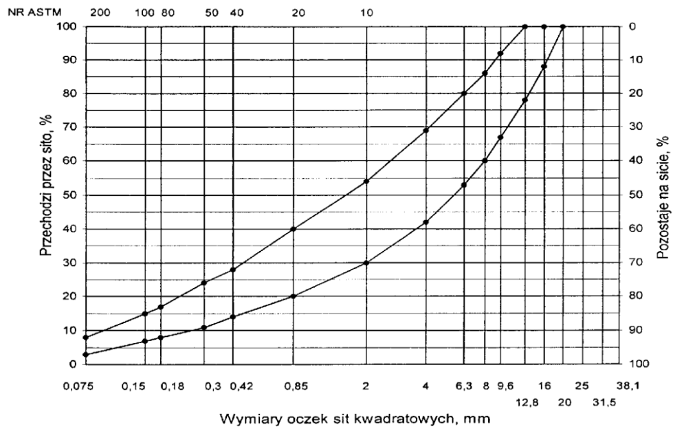
Rys. 9. Krzywe graniczne uziarnienia mieszanki mineralnej BA od 0 do 16 mm do warstwy wiążącej, wyrównawczej i wzmocniającej nawierzchni drogi o obciążeniu ruchem KR1
