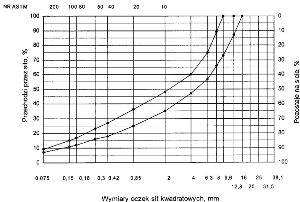
Rys. 7. Krzywe graniczne uziarnienia mieszanki mineralnej BA od 0 do 12,8 mm do warstwy ścieralnej nawierzchni drogi o obciążeniu ruchem od KR4
