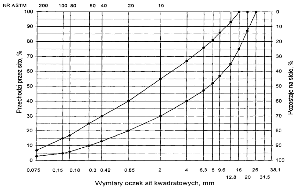
Rys. 8. Krzywe graniczne uziarnienia mieszanki mineralnej BA od 0 do 20 mm do warstwy wiążącej, wyrównawczej i wzmocniającej nawierzchni drogi o obciążeniu ruchem KR1
