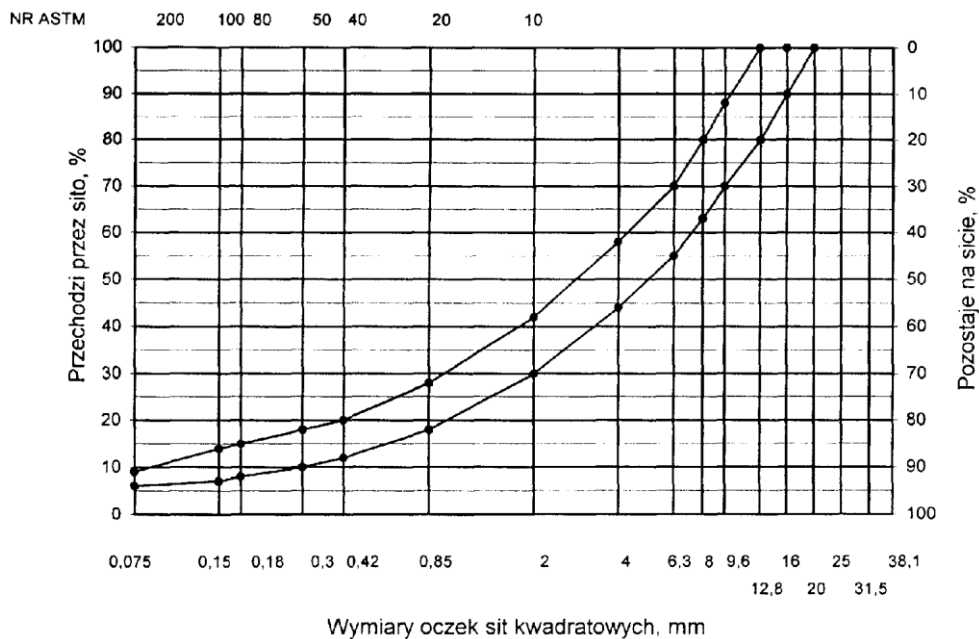
Rys. 6. Krzywe graniczne uziarnienia mieszanki mineralnej BA od 0 do 16 mm do warstwy ścieralnej nawierzchni drogi o obciążeniu ruchem od KR4
