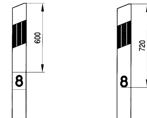
Rys. 8.3.2.2. Umieszczenie znaku hektometrowego U-6 na słupku prowadzącym U-1
