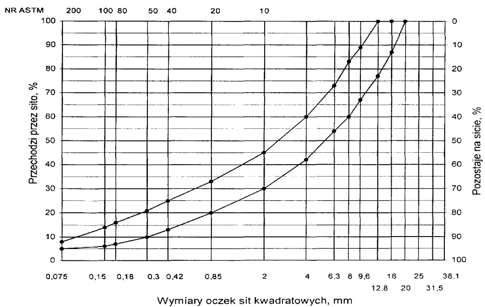
Rys. 13. Krzywe graniczne uziarnienia mieszanki mineralnej BA od 0 do 16 mm do warstwy wyrównawczej nawierzchni drogi o obciążeniu ruchem od KR4
