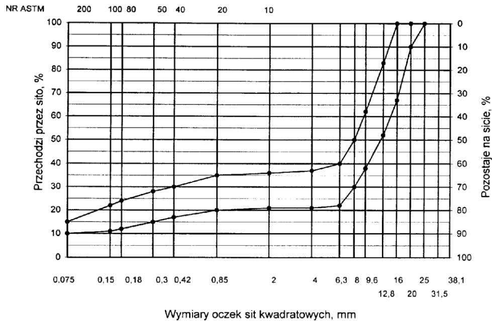
Rys. 5. Krzywe graniczne uziarnienia mieszanki mineralnej BA od 0 do 20 mm (mieszanka o nieciąłym uziarnieniu) do warstwy ścieralnej nawierzchni drogi o obciążeniu ruchem od KR4
