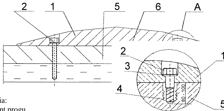
Rys. 4. Przykład umocowania progu do nawierzchni jezdni
