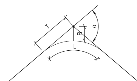
SCHEMAT OZNACZENIA PARAMETRÓW ŁUKÓW
