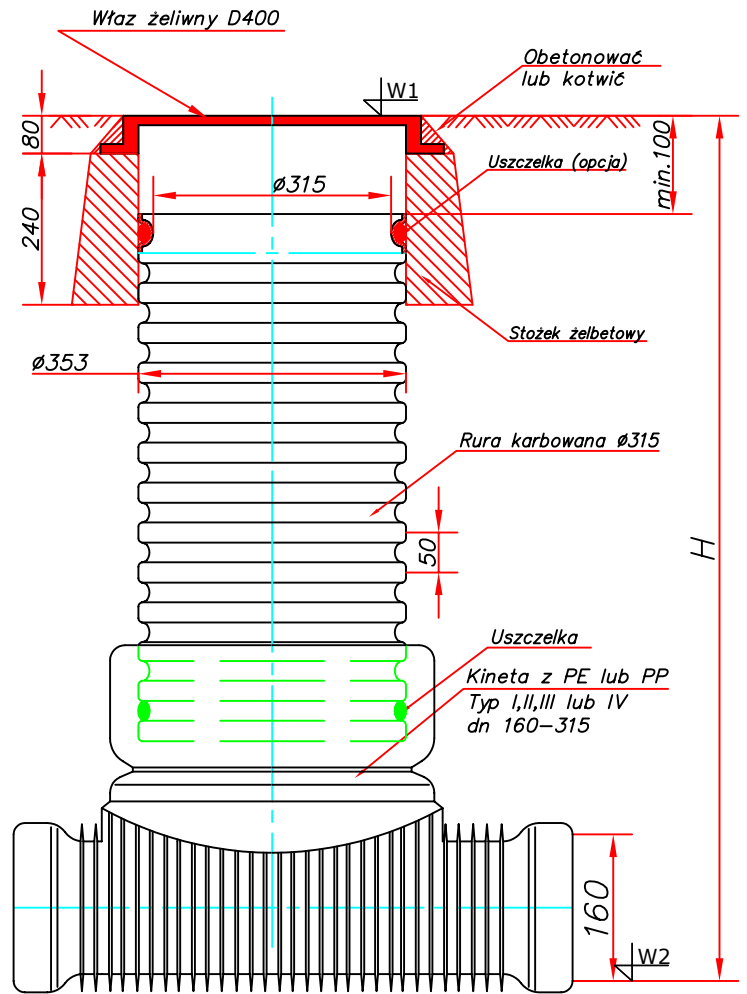
Studzienka inspekcyjna Ø315 na sieci
