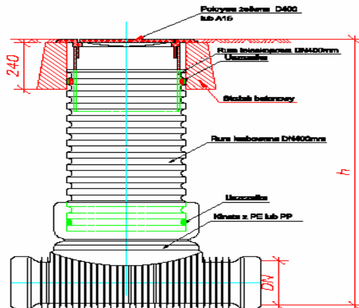
Schemat studzienki \varnothing 315 mm
