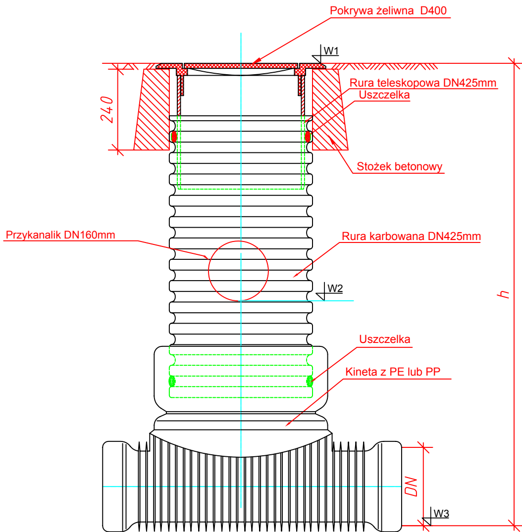
Zestawienie studni Ø425mm na sieci
