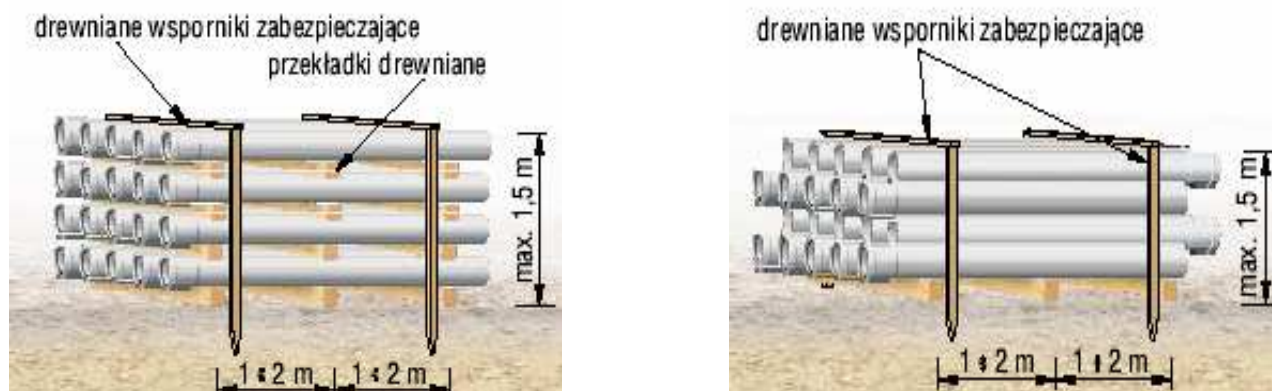
Rysunek poglądowy składowania rur PVC na placu budowy
