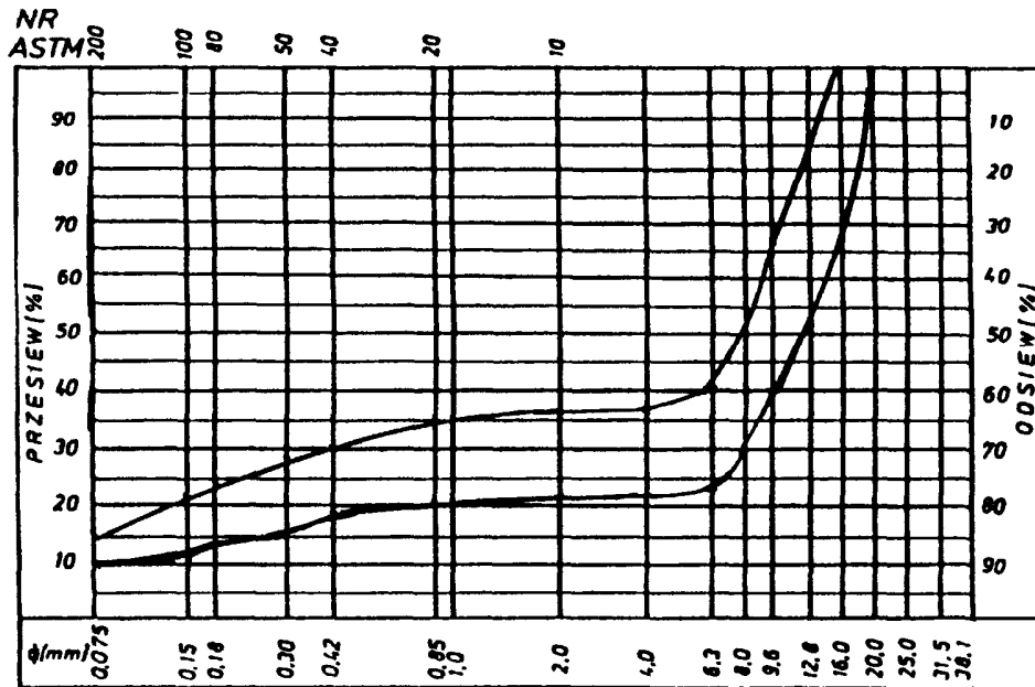
Rys. 5. Krzywe graniczne uziarnienia mieszanki mineralnej 0+20 mm o nieciąglym uziarnieniu do warstwy ściernej z betonu asfaltowego dla KR 3-6
