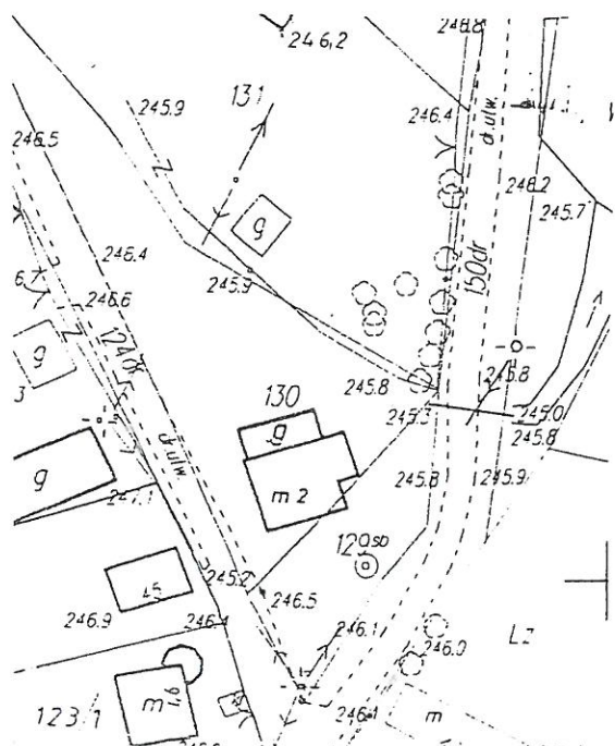
Wyniesienie skala 1 : 1000 y sytuacyjno-wysokościowej
