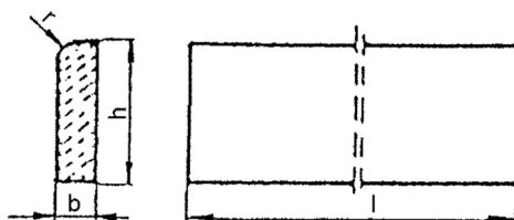
Rysunek 1. Kształt betonowego obrzeża chodnikowego Tabela 1. Wymiary obrzeży
