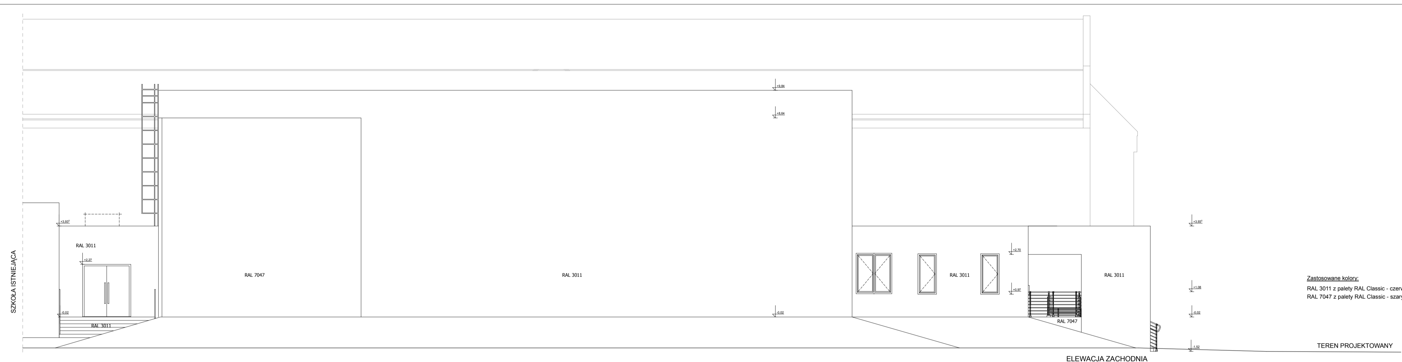
ELEVACJA ZACHODNIA
